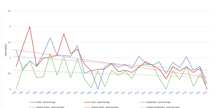
Débit moyen de l'Agly mesuré à Estagel (m 3 /s) et courbes de tendances. Mois juillet, août, septembre 1995-2022 (après mise en eau barrage Agly)
