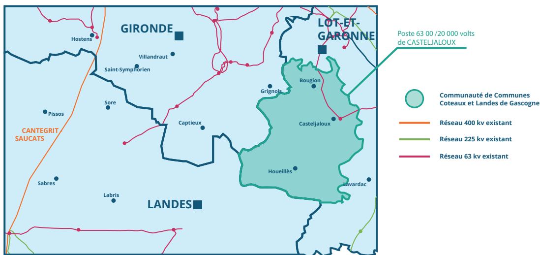
Carte 11. Emplacement poste Casteljalous
