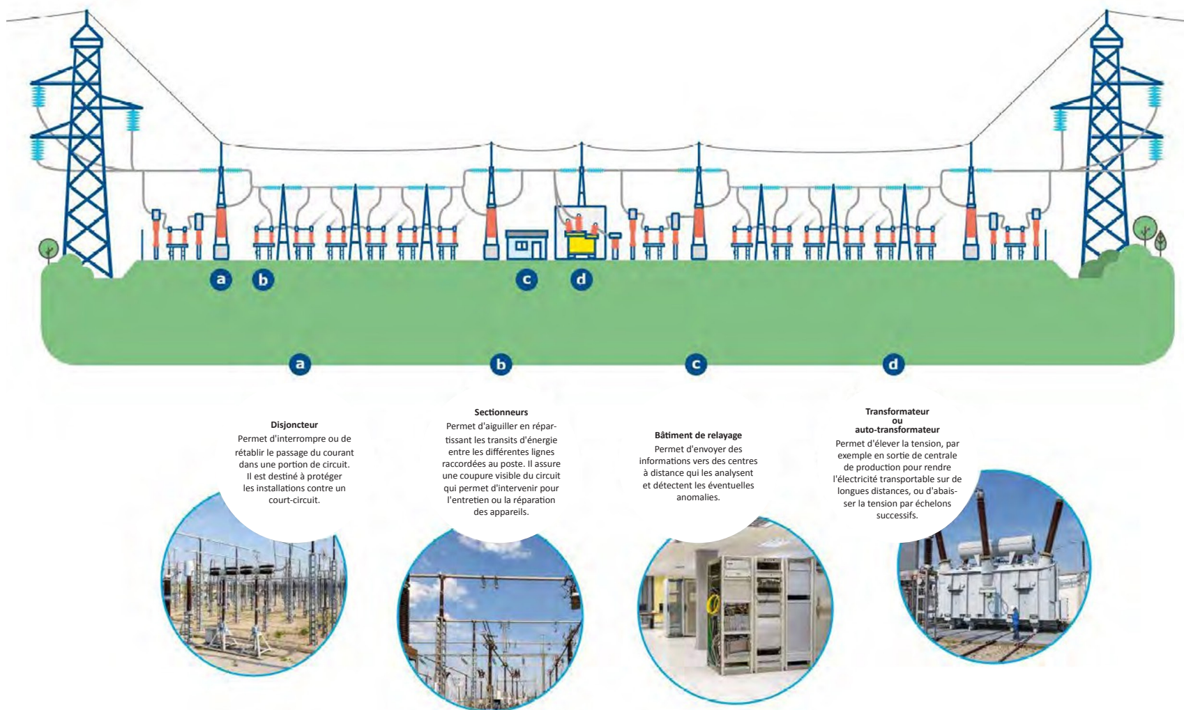
Figure 11. Schéma de principe d'un poste (RTE)
