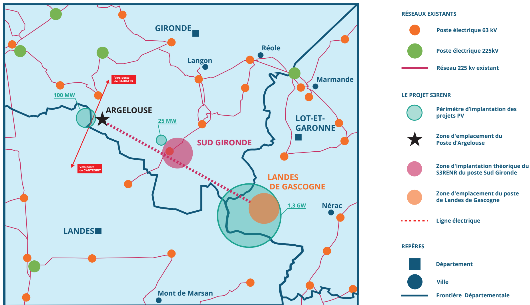
Carte 12 1 . Les postes, la puissance des demandes de raccordement et la ligne
