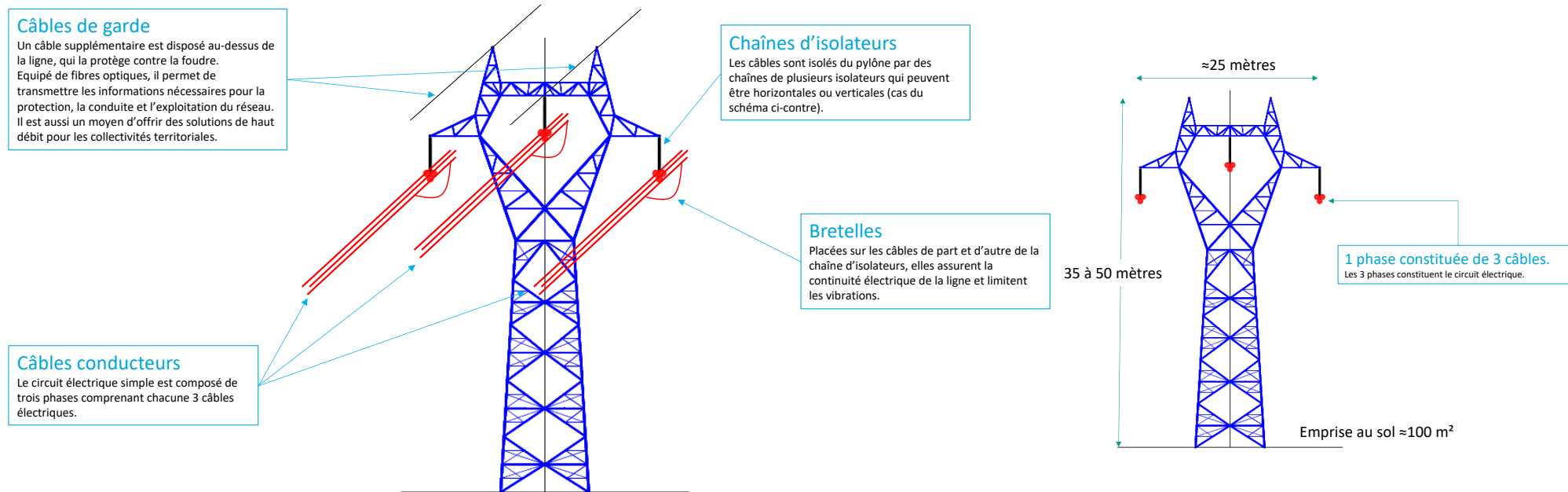
Figure 12. Schéma d'une ligne aérienne à simple circuit (RTE)
