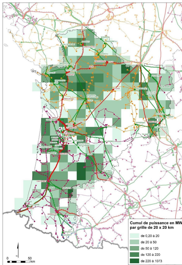
Carte 5. Gisements potentiels de production d'énergies renouvelables (source : S3REnR Nouvelle-Aquitaine)
