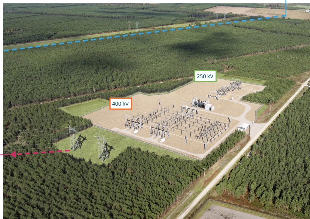
Photo montage du poste d'Argelouse
